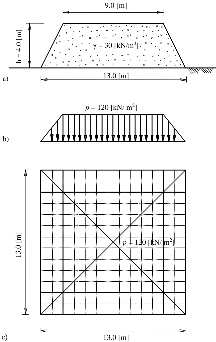
Bild 54 a) Äquivalente Erzmasse b) Belastung c) FE-Netz
