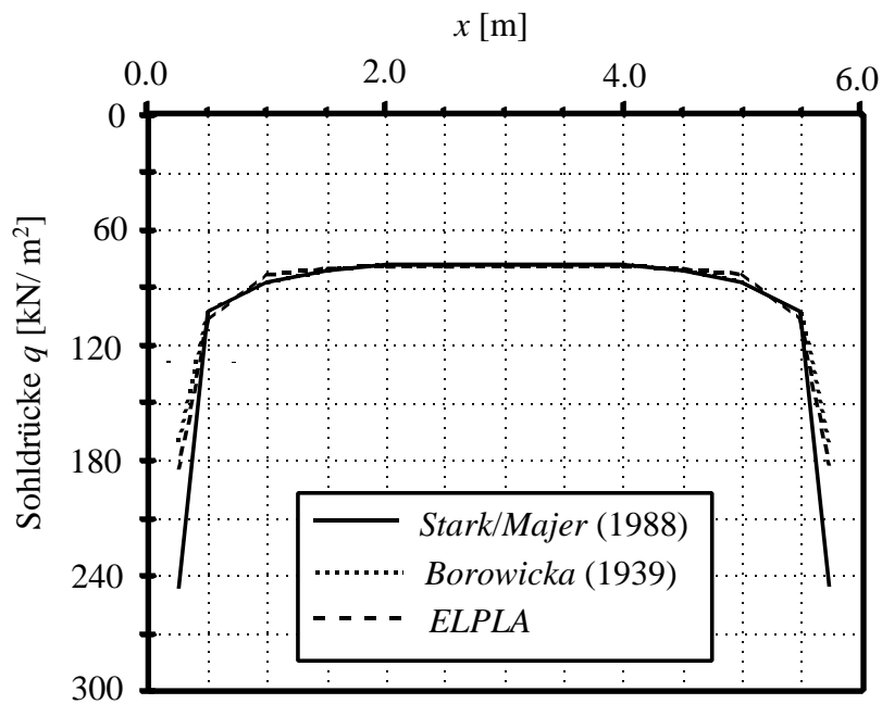
Bild 25 Sohldruckverteilung q [kN/m 2 ] im Schnitt a-a, k_B = \pi/30 , d = 18.5 [cm]
