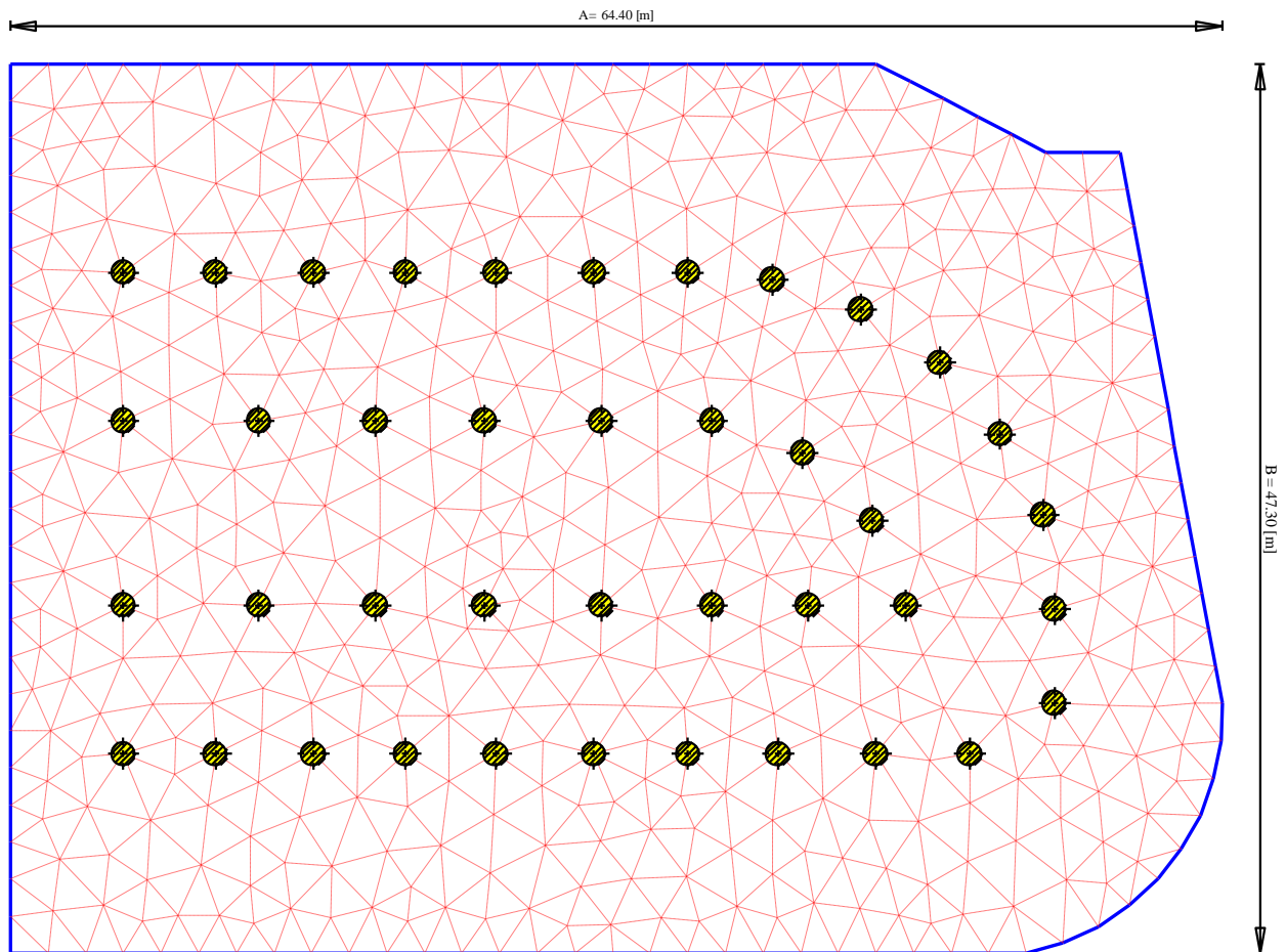
Bild 5-3 Netz der Pfahlplatte des Westend 1 mit Pfählen
